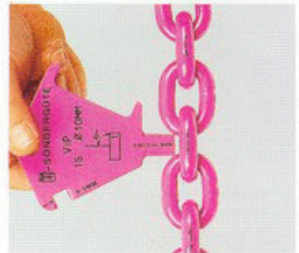
Prüfen Teilungs-Verlängerung durch Nenndicken-Verschleiß
